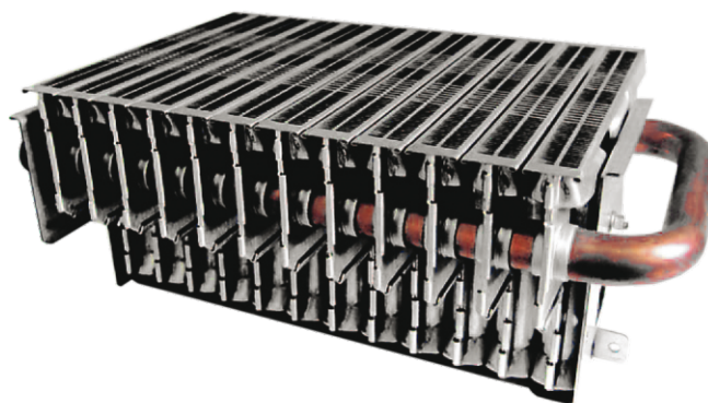
Arzător Low NOx - răcit cu apă
