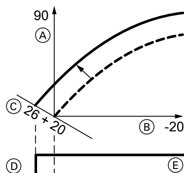
Fig. 47 Exemplul 1: Modificarea valorii nominale a temperaturii de ambianță de la 20 la 26 °C
